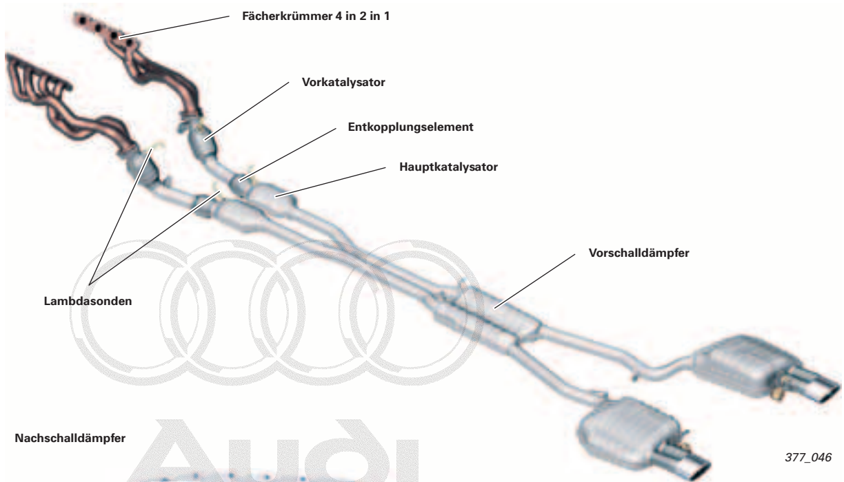
Abgasanlage RS4
