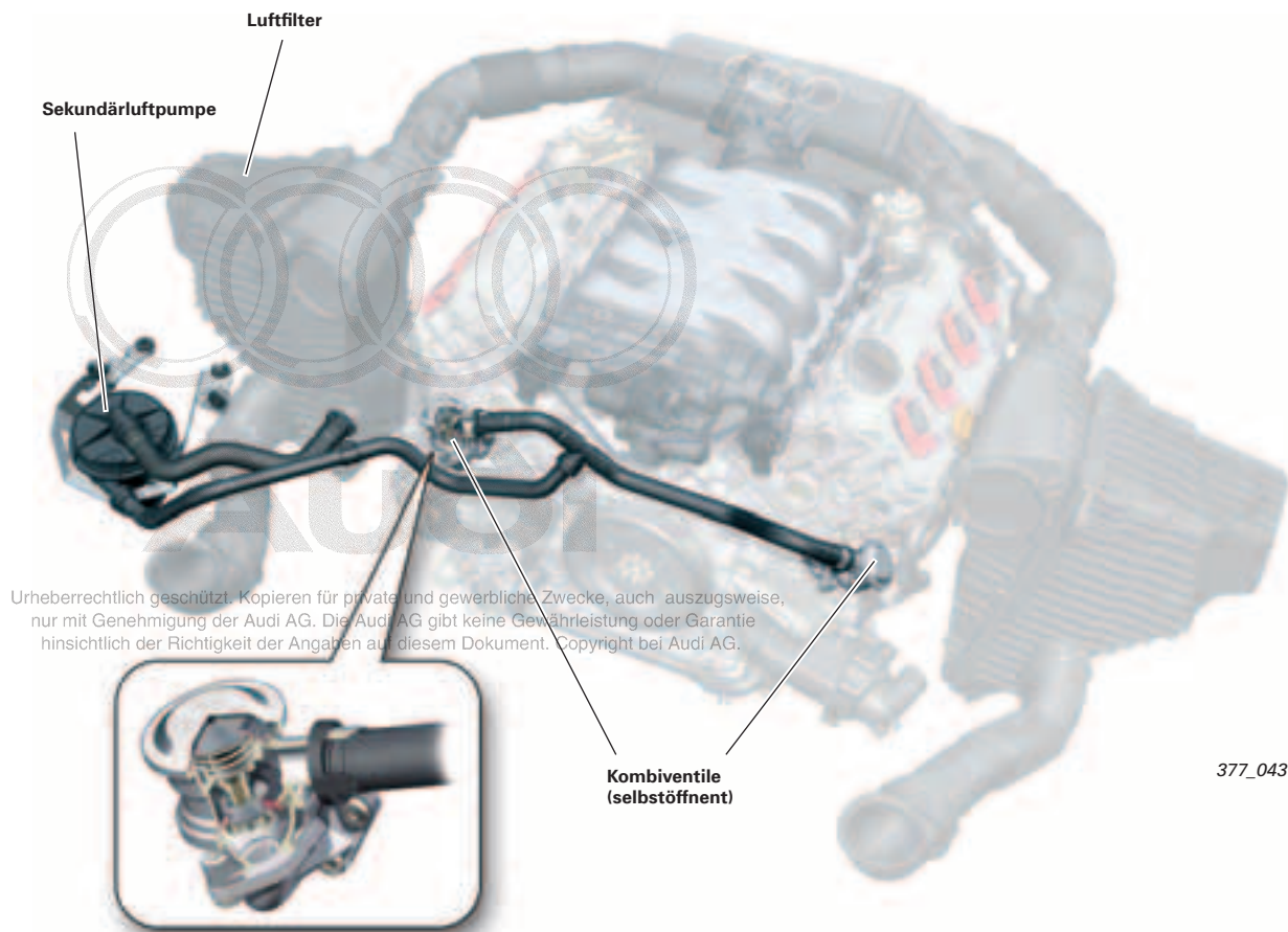
Sekundärluftsystem Q7
